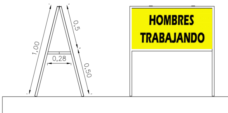
VISTA LATERAL
