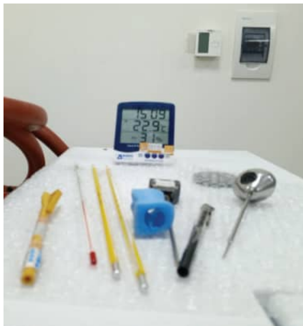
Variedad de termómetros en proceso de calibración
